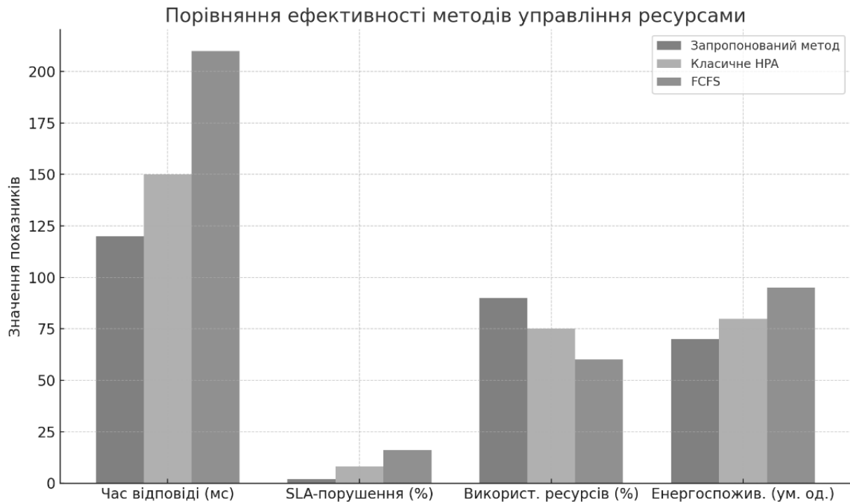
Рис. 1. Порівняльна ефективність методів управління ресурсами у хмарному середовищі Comparative efficiency of resource management methods in the cloud environment
